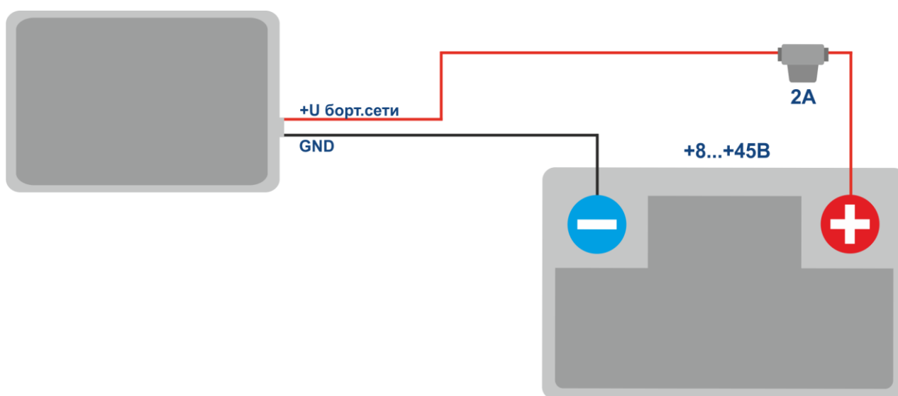
Рисунок 3 - Типовая схема подключения питания терминала
