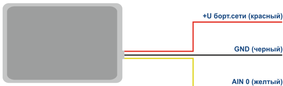
Рисунок 2 – Цветовая маркировка проводов терминала
